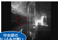
※粒子画像流速測定法(Particle Image Velocimetry)による流れを見える化した画像
