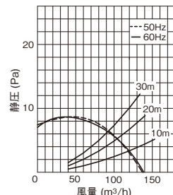
●VFP-12WSs 静圧-風量特性 抵抗曲線は塩ビVP管φ150の場合
