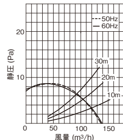
●VFP-12WSSs 静圧-風量特性 抵抗曲線は塩ビVP管φ150の場合
