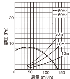
●VFP-12Ws 静圧-風量特性 抵抗曲線は塩ビVP管φ150の場合
